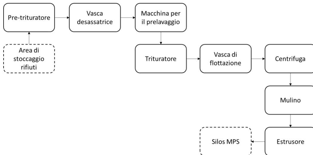
Figura 1 –Schema a blocchi processo di trattamento rifiuti.
